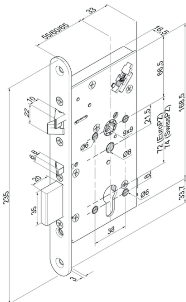
Maßzeichnung Vollblatt
